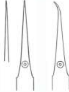
FO-608-12 FO-609-12 12 cm/4¾" 12 cm/4¾" 0,3 mm 0,3 mm
