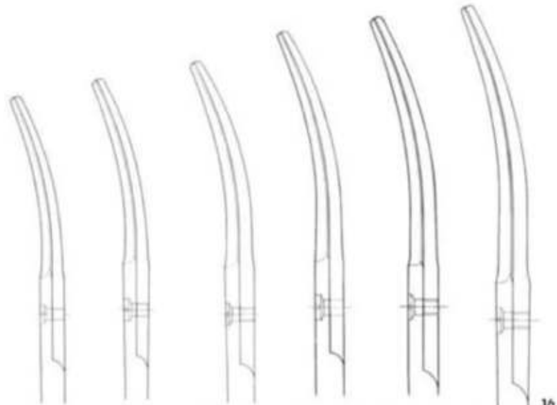
MA 101-11 11.5 cm MA 101-13 13 cm MA 101-14 14.5 cm MA 101-15 15 cm MA 101-16 16.5 cm MA 101-17 17.5 cm
